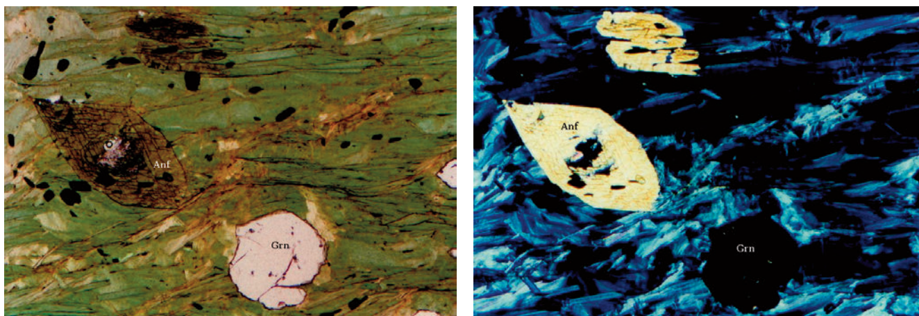
Fig. 1. Microstruttura del campione di pietra ollare US596 al microscopio polarizzatore in luce trasmessa: a) luce non polarizzata, b) luce polarizzata. Spiccano sulla massa di fondo un porfiroblasto di anfibolo (Anf) e un granulo di granato (Grn).
